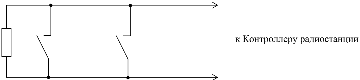
Рисунок 3. Подключение датчиков с нормально разомкнутыми контактами (режим работы 1).
